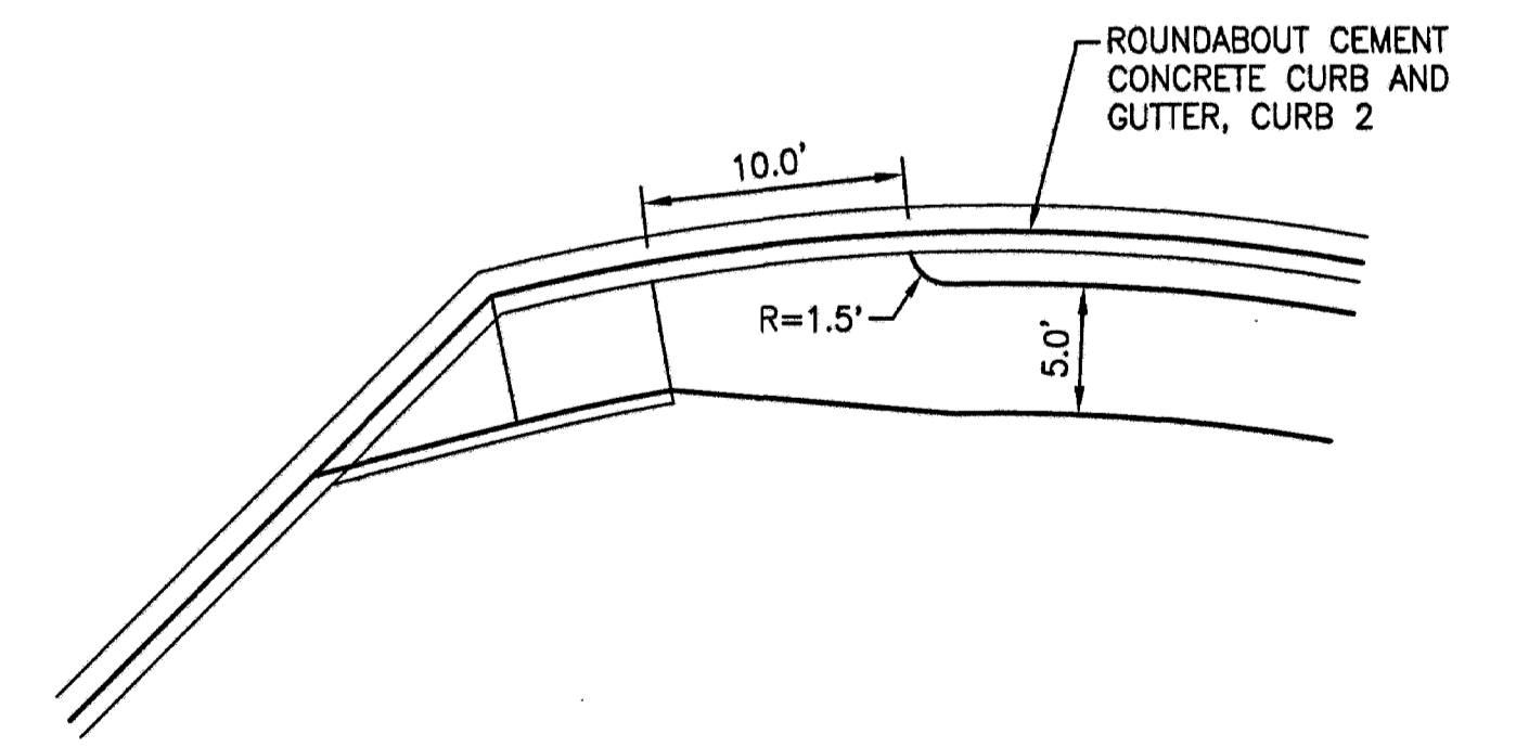
PLAN VIEW - STA 173+21.4
