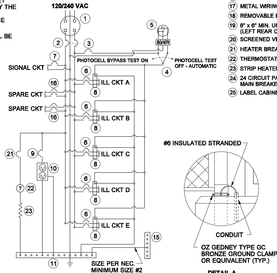
WIRING SCHEMATIC
